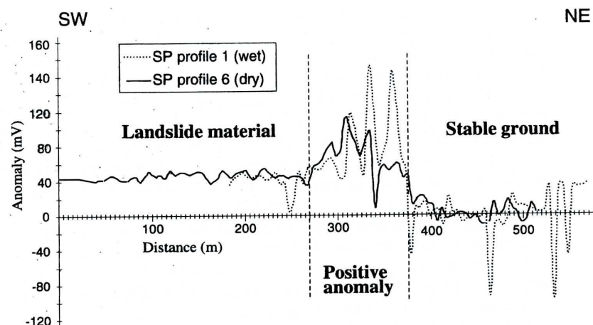
FIG. 3.3 – Mesure de PS effectuée sur le mouvement de Boud (Suisse), d'après Bruno et Marillier (2000)
