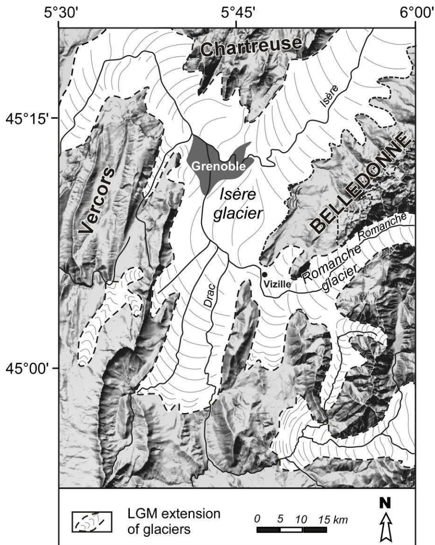
Fig. 3-4: Dernière extension maximale des glaciers (LGM) au Würm sur fond de MNT IGN au pas de 50 m. D'après Montjuvent (1978).
