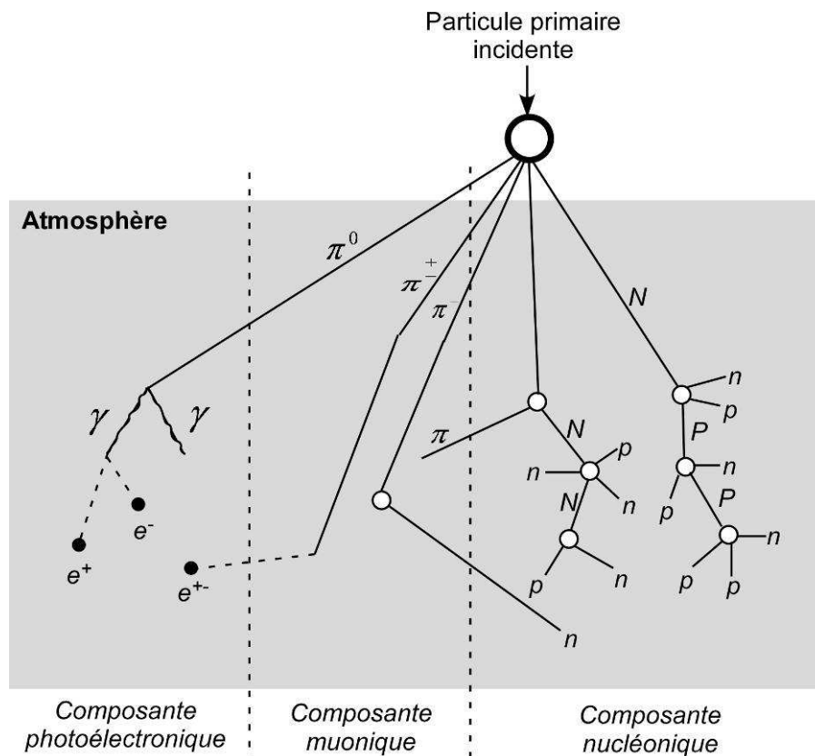
Fig. 8-1 : Représentation schématique de la cascade nucléaire issue de l'interaction des particules très énergétiques du rayonnement cosmique primaire avec les constituants de l'atmosphère terrestre pour former les particules secondaires : N, P : neutrons et protons de haute énergie ; n, p : neutrons et protons thermiques ; \pi, \mu : muons ; \gamma, e^+, e^- : rayons gamma, positrons, électrons (Siame et al., 2000).
