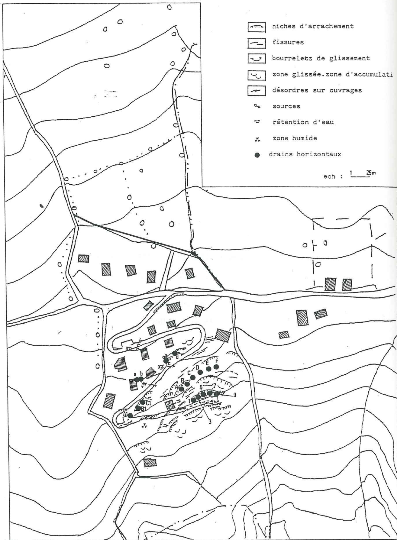
LOCALISATION DES DRAINS SUBHORIZONTAUX PAR RAPPORT AUX MANIFESTATIONS D'INSTABILITE RELEVES SUR LE LOTISSEMENT
