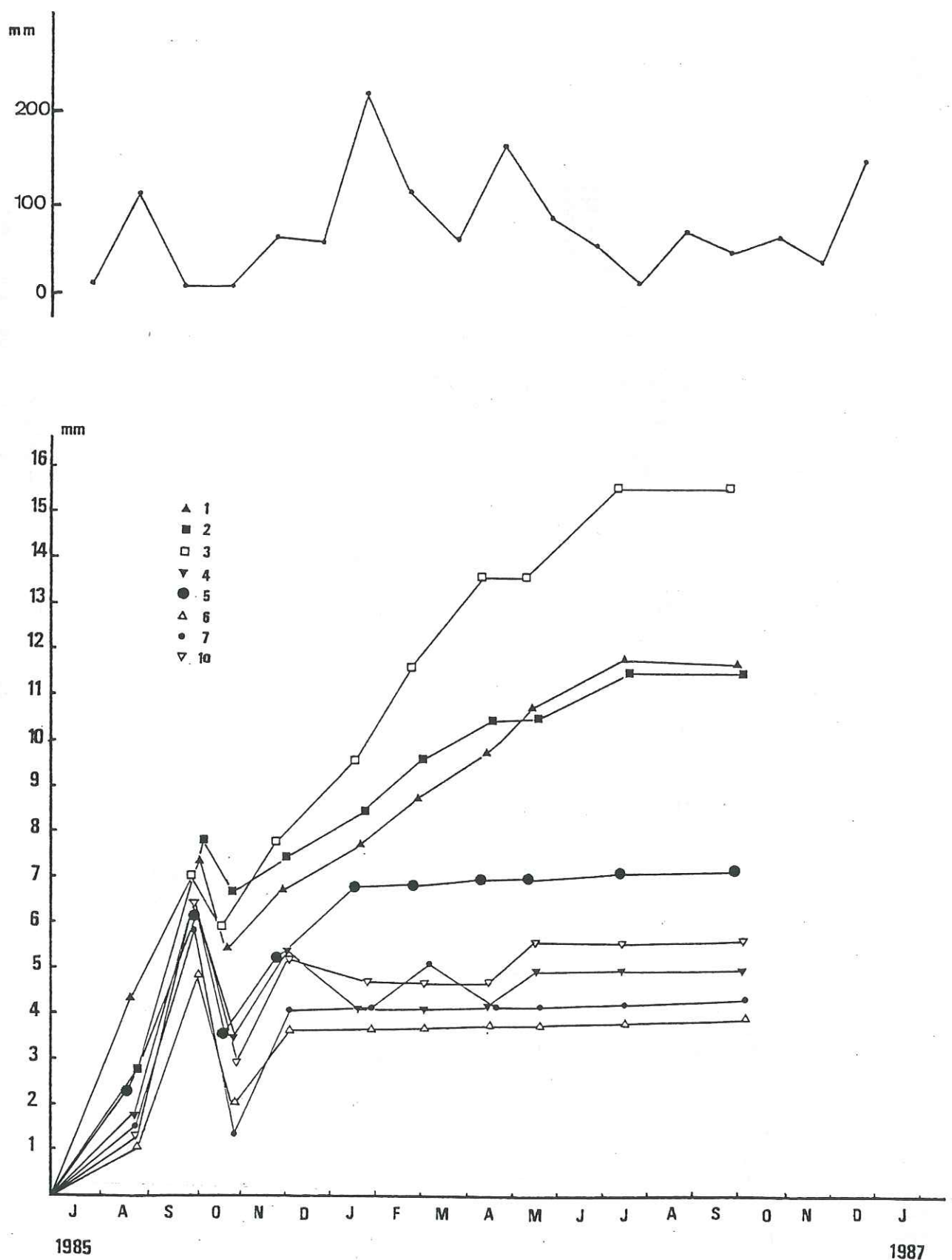
figure 27 : REPRESENTATION DES DEPLACEMENTS CUMULES DES REPERES TOPOGRAPHIQUES DU LOTISSEMENT EN FONCTION DU TEMPS et COMPARAISON DE CES DEPLACEMENTS AVEC LES RELEVES PLUVIOMETRIQUES
