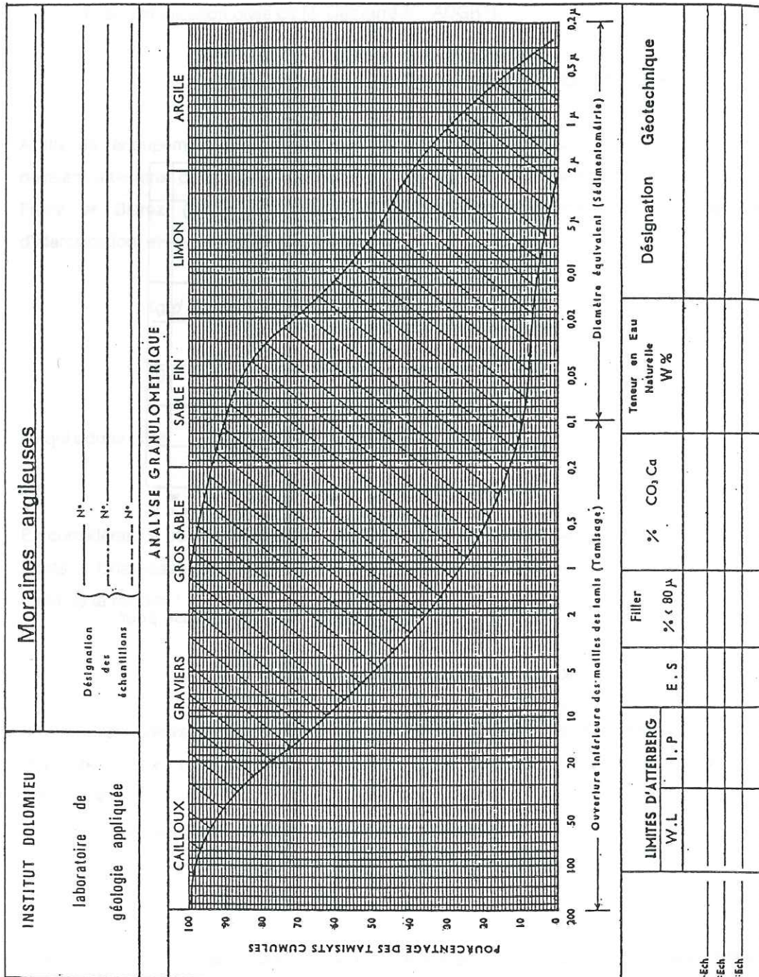
figure 54 - Fuseau granulométrique des moraines argileuses
